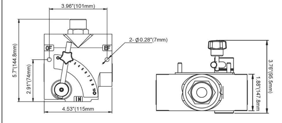
DIMENSION D'INSTALLATION INSTALLING DIMENSION
