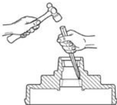
*Technique d'enlèvement de la bague de roulement
